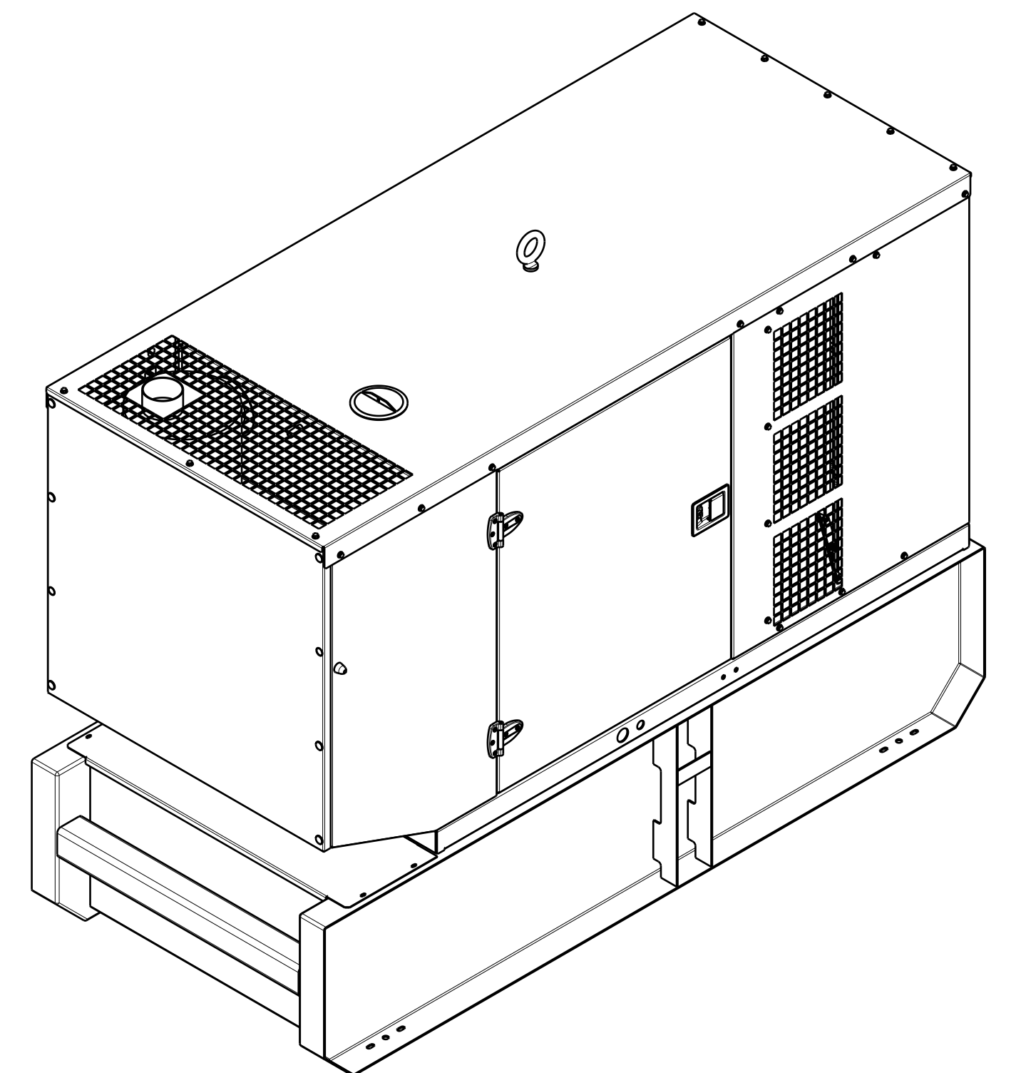
Vue isométrique Echelle : 1:15
